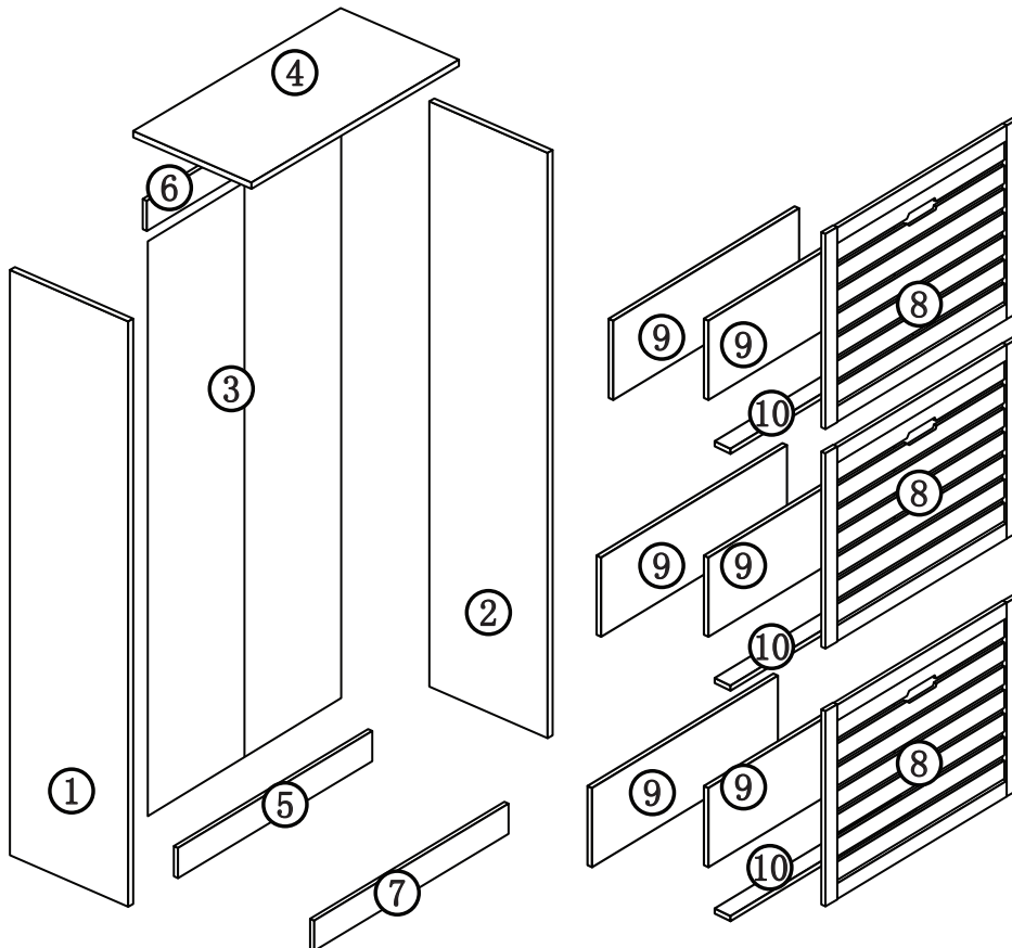
⑨ 484x137x12mm
